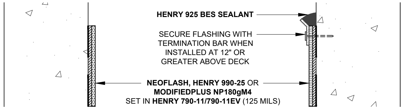
MOP-GRADE FLASHING N.T.S
