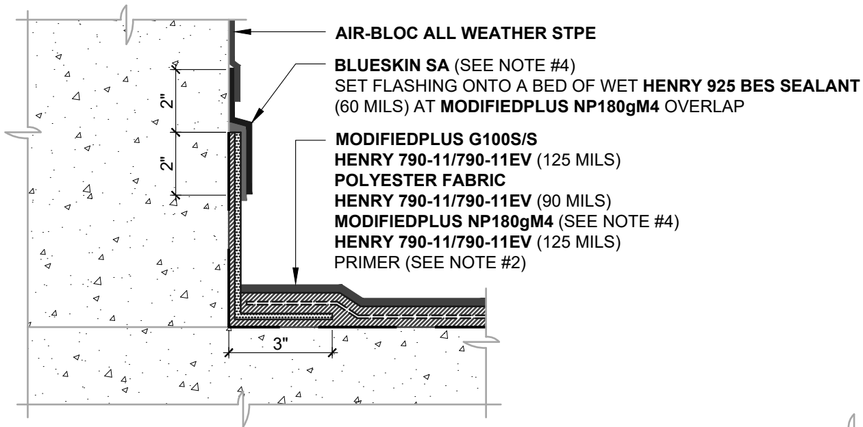
MOP-GRADE FLASHING N.T.S
